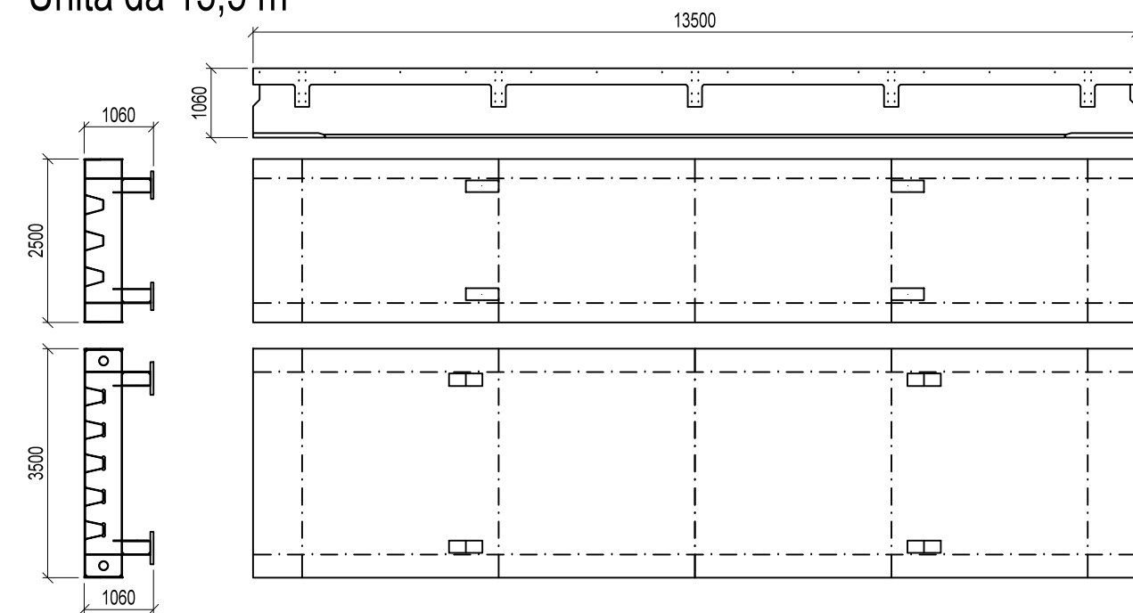
Unità da 13,5 m
