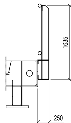
Parapetto pedonale
