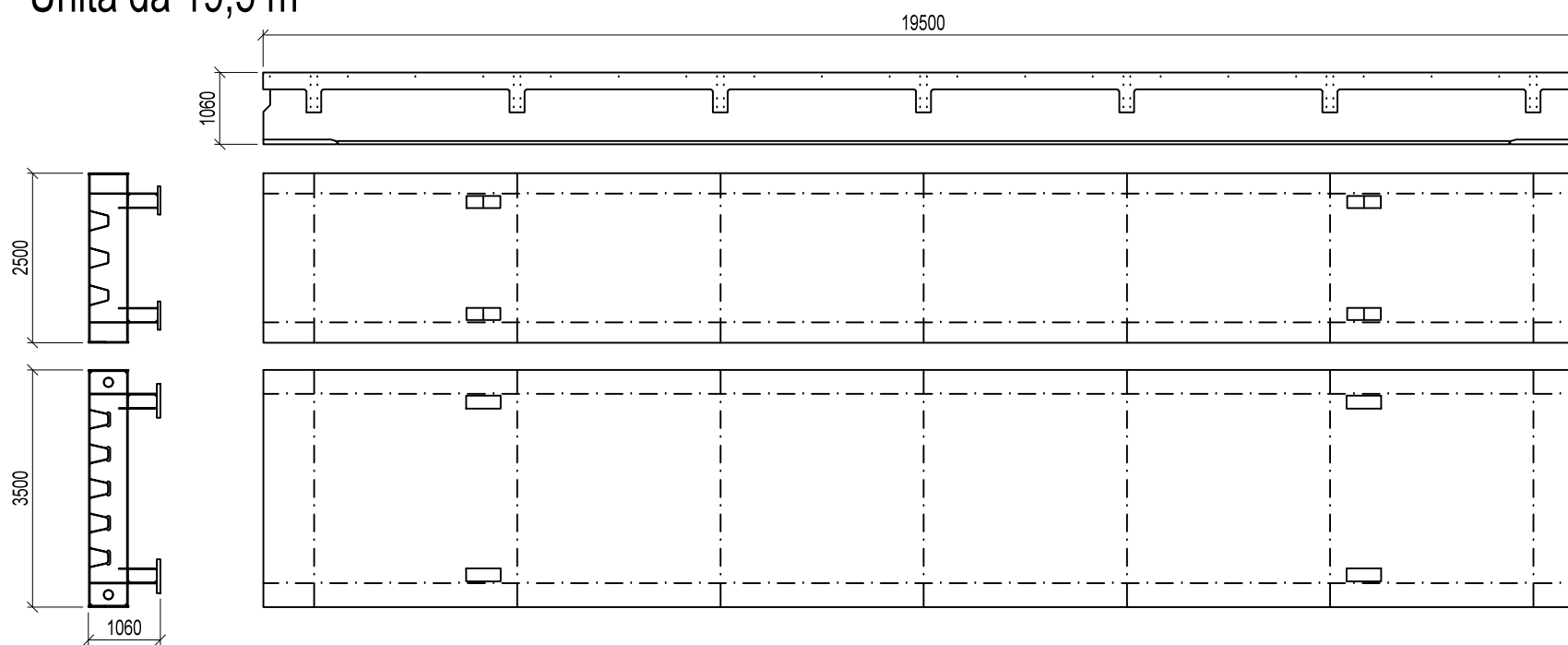
Unità da 19,5 m
