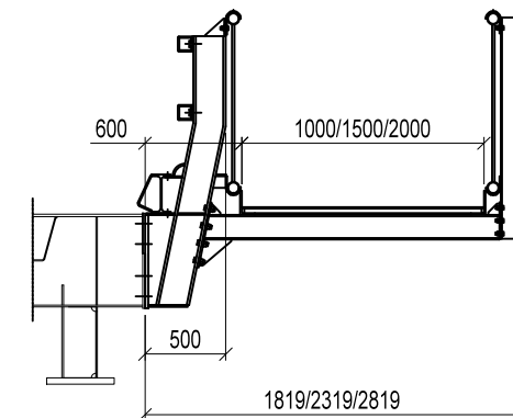
Passerella pedonale esterna
